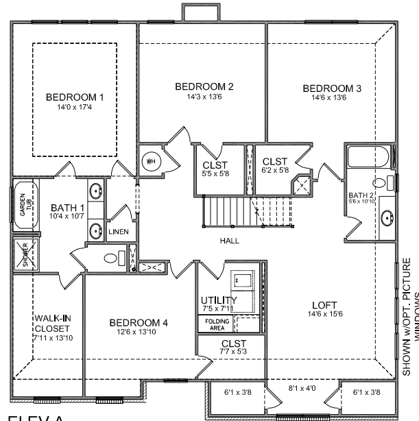
ELEV A
