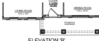
ELEVATION 'B'
