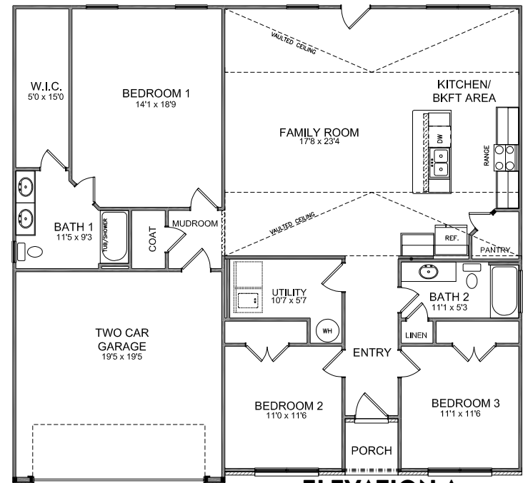
ELEVATION A
